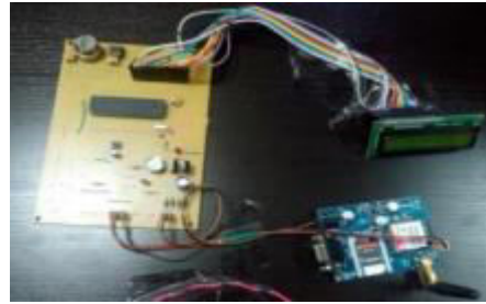
Fig.1. Hardware module.
